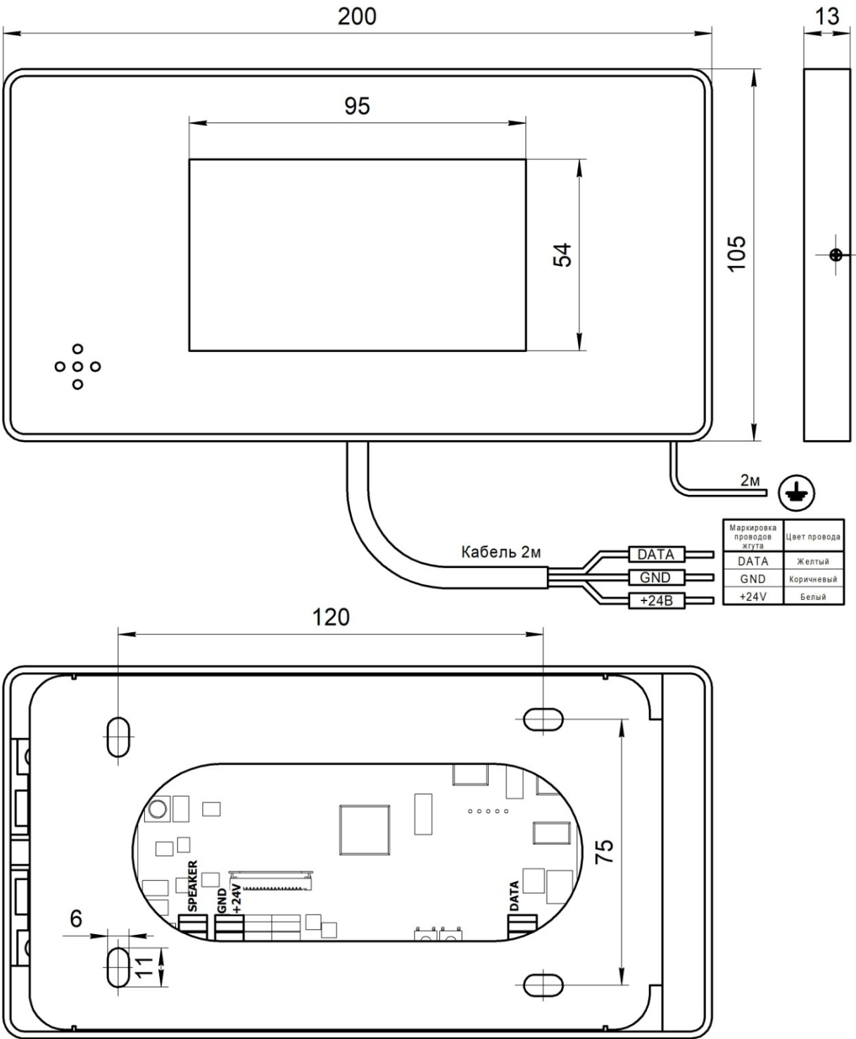
Рис.1 Внешний вид Табло накладное МАЛАХИТ НШЕК.468232.132-01
